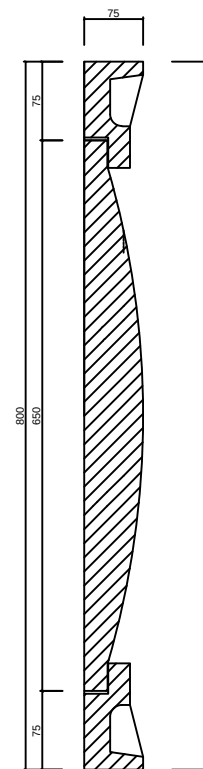
Mặt cắt 1-1
