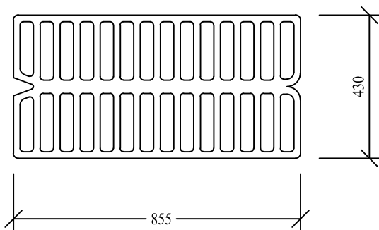
Mặt bằng
